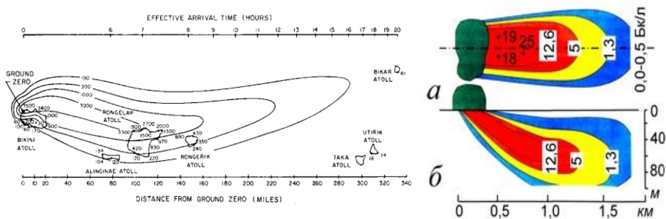
Рисунок 4.4. Зона загрязнения, возникшая в результате испытаний термоядерного устройства (взрыв Коста-Браво) на атолле Бикини 1954 г. по данным
