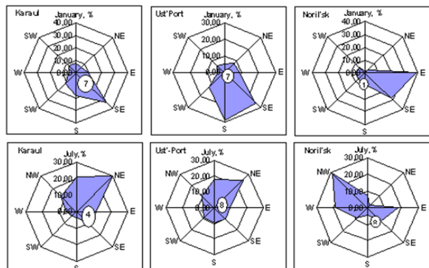
Рисунок 4.22. Роза ветров Норильска, Усть Порты и пос. Караула в январе и июле [по Соломатину и др., 1989; цит по ESTABLISH, 2002]
