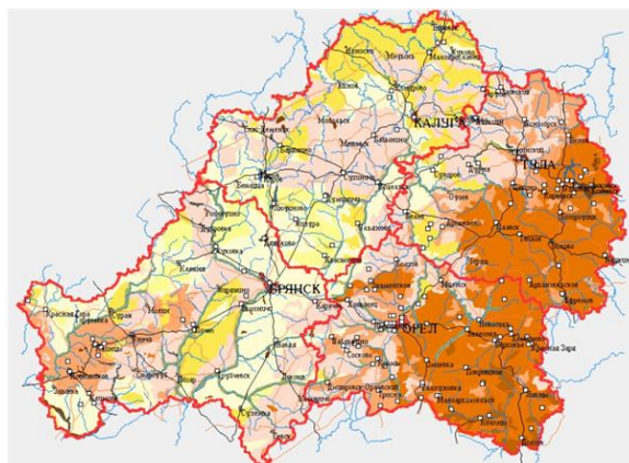
Рисунок 5.3. Карта йодного статуса 4-х областей России, пострадавших в результате аварии на ЧАЭС 1986 г (Выделены населенные пункты, для которых проводились картографические расчеты по международному проекту
